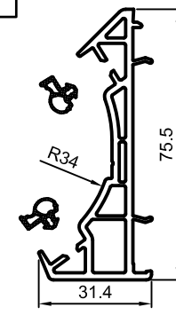
NP0150 Адаптер Упорное уплотн. DP2440
