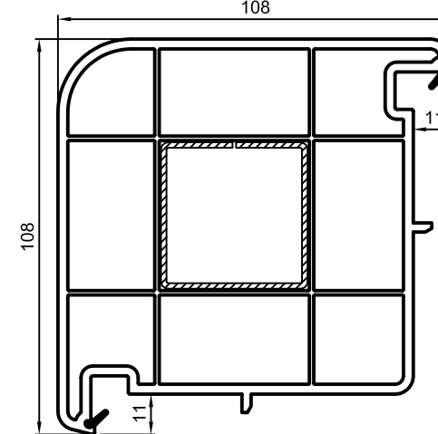
NP0100 Угл. соединитель 90° Сталь: 40/40/1,5 715303
