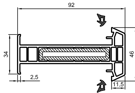
NP0130 Сталь: 10x60x2,9 VS0130 Клинов. уплотнение DP0130
