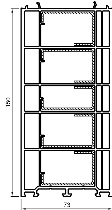
NP3300 Сталь: 16/26,6/42/8/1,5 возможно VS1020 Сталь: 16/26,6/42/8/1,25 возможно VS1120 Сталь: 16/18,6/42/8/1,5 возможно VS1010
