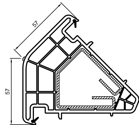
416240 Угл. соединитель на 135° Сталь: 50/30,7/30,7/50/2,0 415140
