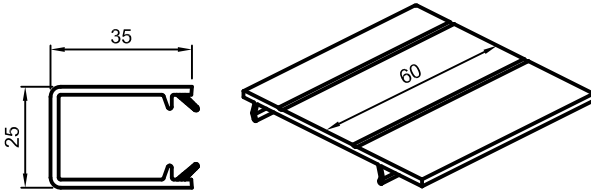
MT0140 Дистанционная вставка для VS0140
