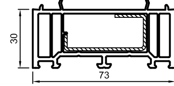
NP1350 Сталь: 16/18,6/42/8/1,5 возможно VS1010
