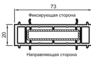
NP0120 Сталь: 10x50x1,5 405015
