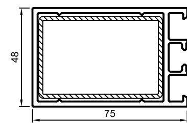
416269 Сталь: 40/60/2,0 AR4630 Нипельный шуруп 407900
