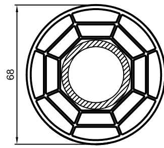
NP0160 ПВХ-труба Ø68 Сталь: Ø33,7/3,2 415016
