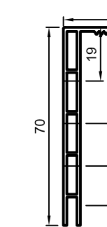
ZF2020 для рам HP1100, HP2100, HP2110
