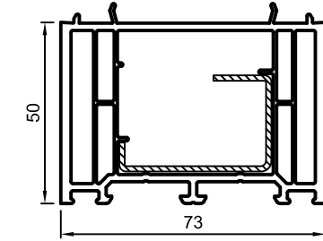
NP1550 Сталь: 16/26,6/42/8/1,5 возможно VS1020 Сталь: 16/26,6/42/8/1,25 возможно VS1120
