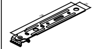
MT1000 Монтажный анкер
