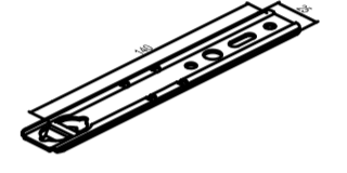
MT1010 Поворотный монтажный анкер
