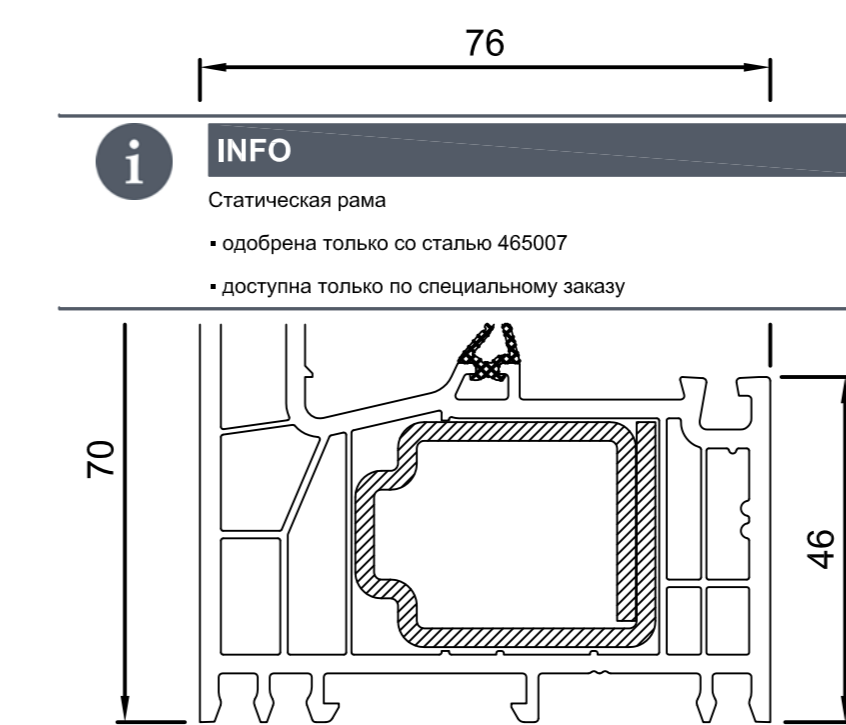
760010 (A) Сталь: 40x30 465007
