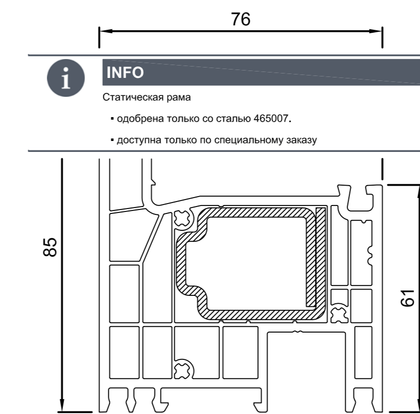
760013 (A) Сталь: 40x30 465007
